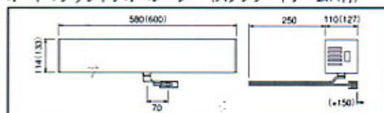
オートマチックドアオペレーター（スタンダードアームA付）
